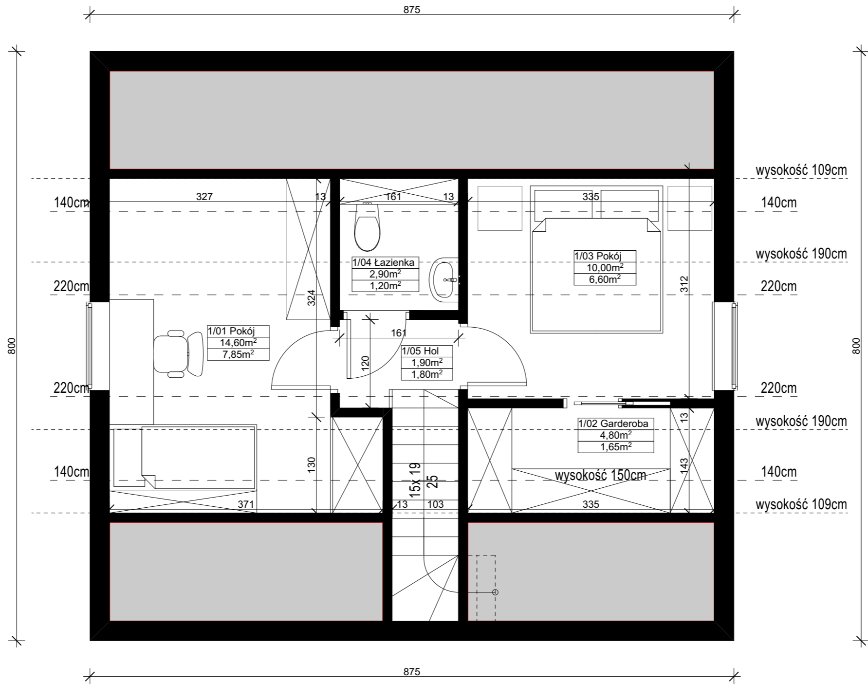
Przykładowa aranżacja układu funkcjonalnego.
